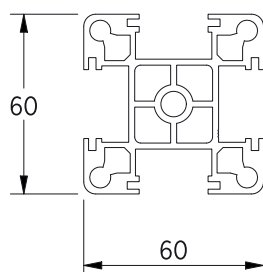
PROFILO PIANTONE SP001
