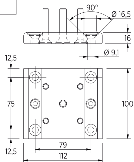
ALTERNATIVA CON SUPPORTO FRONTE SOLETTA SP111 SLAB-FRONT SUPPORT SP111
