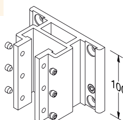
ALTERNATIVA CON SUPPORTO FRONTE SOLETTA SP111 SLAB-FRONT SUPPORT SP111
