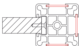
PROFILO 30x2 SP005 per chiudere le vie inutilizzate for closing unused slots
