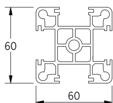
PROFILO PIANTONE SP001
